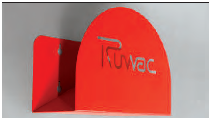
Schlauchhalter, Stahlblech, pulverbeschichtet, rot, Montage an der Wand L - 330 mm, B - 123 mm, H - 238 mm, incl. Befestigungsmaterial Art-Nr: 12080
