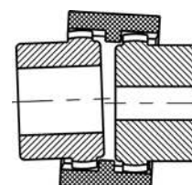
Verlagerung winklig-radial Misalignment angular-radial
